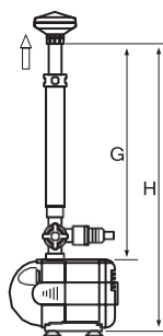
Рис.2. Высота насосов
