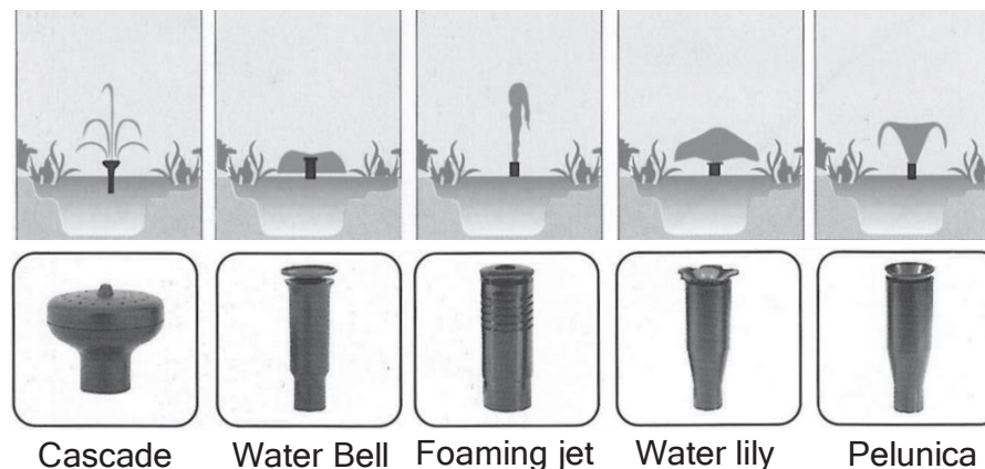
Рис. 1. Дополнительные форсунки.
