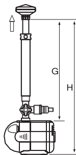
Рис.2. Висота насосів
